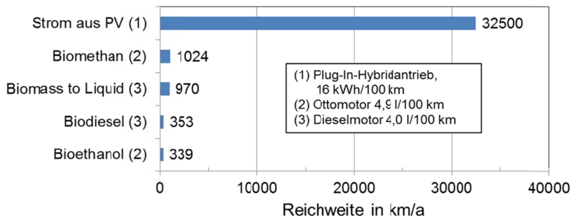
Abbildung 37: Fahrzeugreichweite mit dem Jahresertrag von 1 a = 100 m 2 Energiepflanzenanbau (2,3) und von 40 m 2 PV-Modulen, aufgeständert auf 100 m 2 ebener Grundfläche, Quellen: Photon, April 2007 (1) und Fachagentur Nachwachsende Rohstoffe (2), (3)
