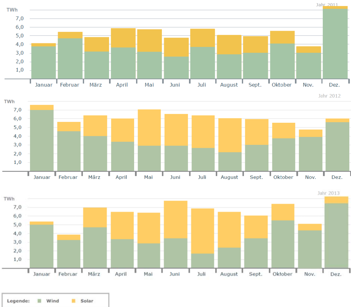
Abbildung 34: Monatliche PV- und Windstromproduktion der Jahre 2011-2013 [ISE4]
