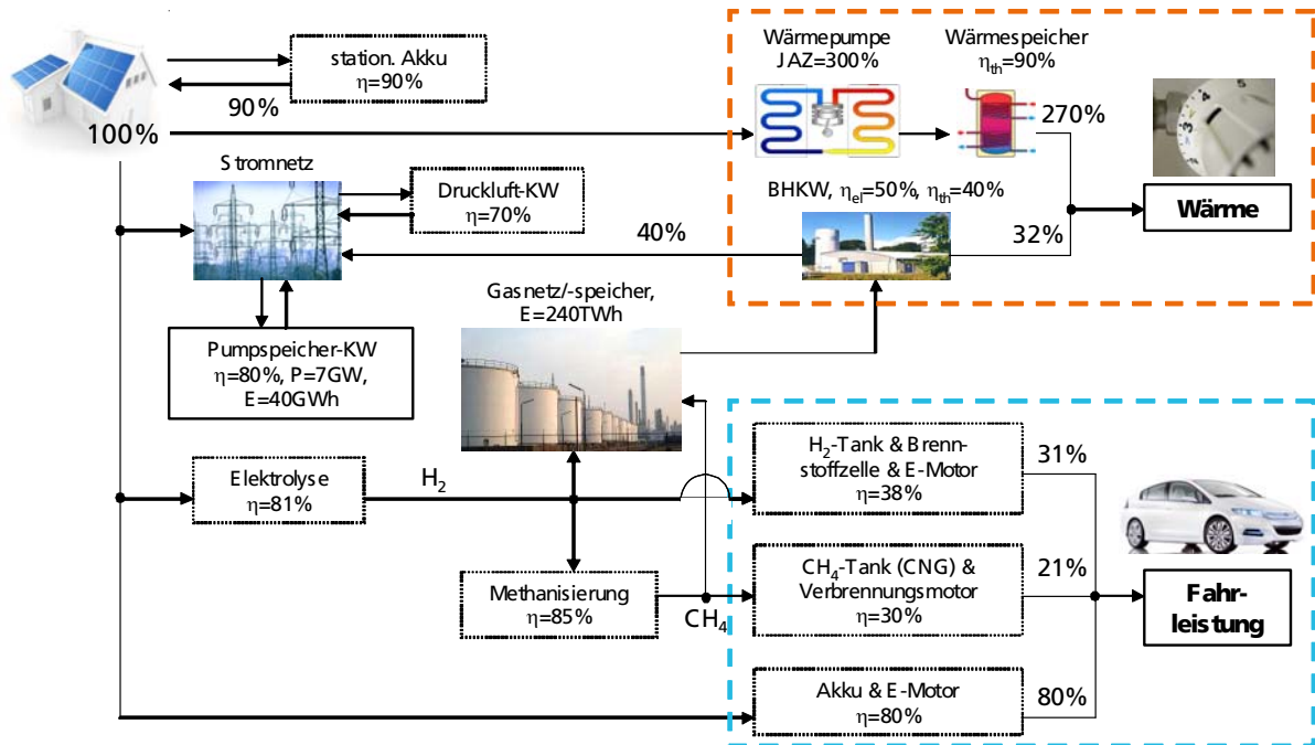
Abbildung 64: Mögliche Pfade zur Wandlung und Speicherung von PV-Strom mit orientierenden Angaben zu Wirkungsgraden
