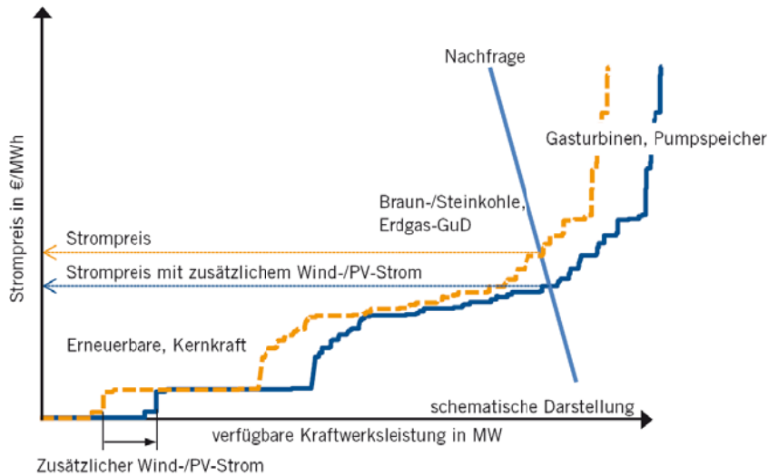
Abbildung 8: Einfluss von EE auf die Preisbildung an der Strombörse [WEC]
