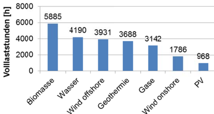
Abbildung 38: Prognostizierte Vollbenutzungsstunden für ganzjährig betriebene Anlagen, gemittelte Werte für die Jahre 2012 bis 2016, Daten aus [R2B]
