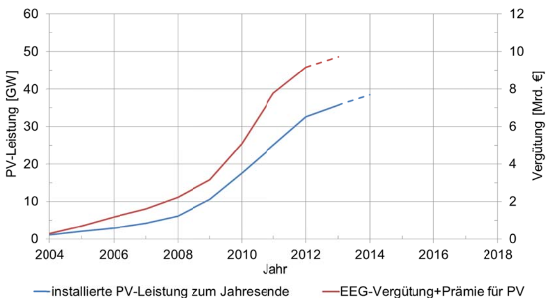
Abbildung 6: PV-Ausbau und Vergütungssumme, Zahlen aus [BMWi1], den Jahresabrechnungen der Netzbetreiber und Schätzungen
