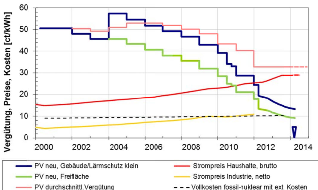
Abbildung 5: EEG-Vergütung von PV-Strom nach dem Datum der Inbetriebnahme für neue Anlagen, durchschnittliche EEG-Vergütung von PV-Strom für Anlagenbestand (Quotient aus der Vergütungssumme lt. Abrechnung Netzbetreiber und der gesamten PV-Stromproduktion, teilw. geschätzt), Vollkosten der fossil-nuklearen Stromerzeugung [IFNE], Strompreise aus [BMW1], teilw. geschätzt
