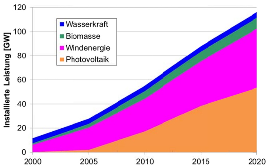
Abbildung 45: Szenario „2011 A“ für den Ausbau von EE-Stromleistung, Daten aus [IFNE]
