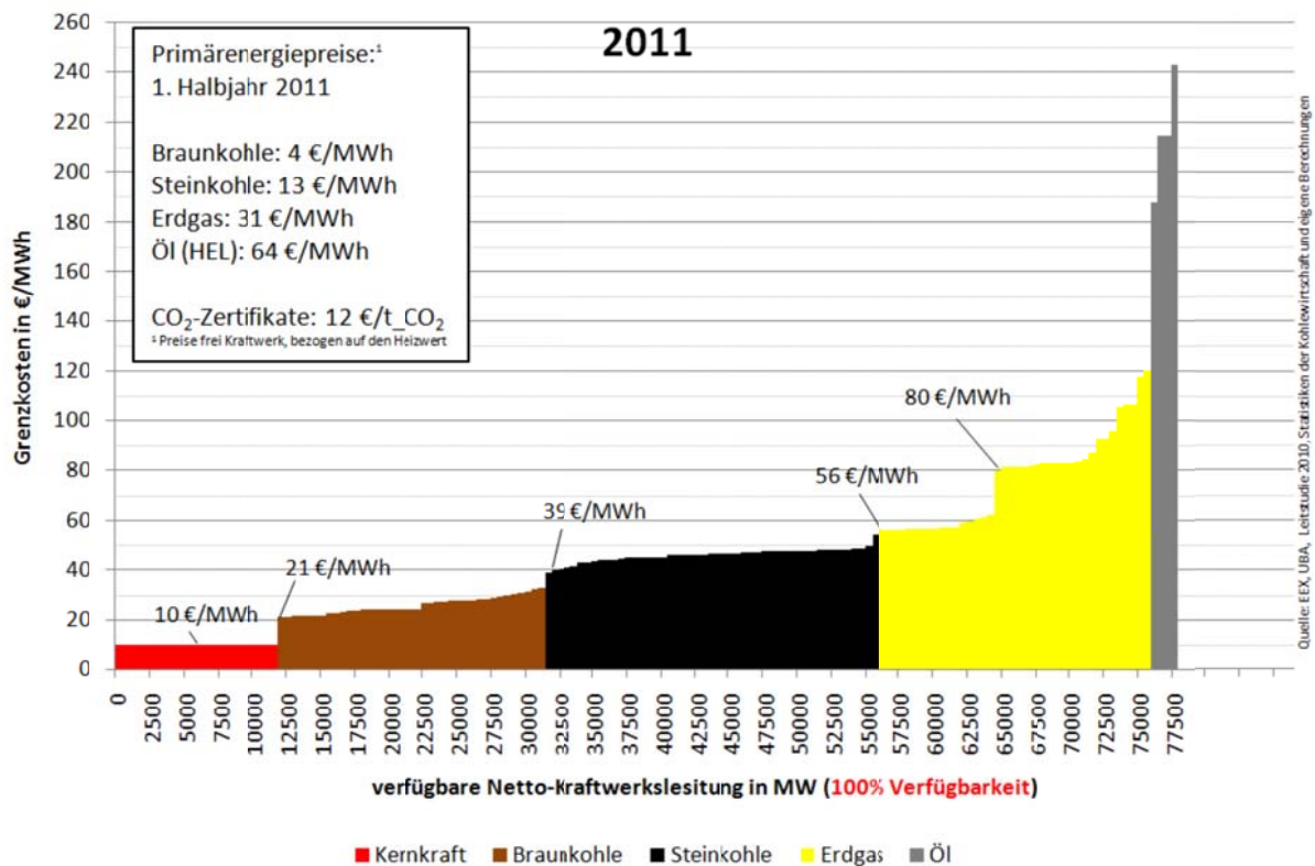
Abbildung 10: Merit Order der konventionellen Kraftwerke 2011 [IZES]; die Angaben zu Primärenergiepreisen beziehen sich auf Brennwerte, die Grenzkosten auf elektrische Energie
