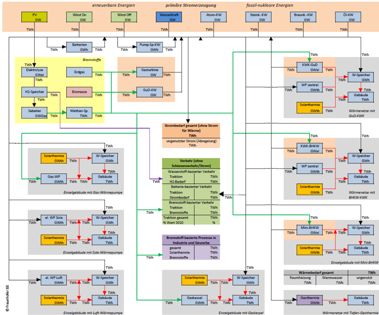
Abbildung 46: Szenario eines deutschen Energiesystems, schematische Darstellung der Systemzusammensetzung. [ISE5]
