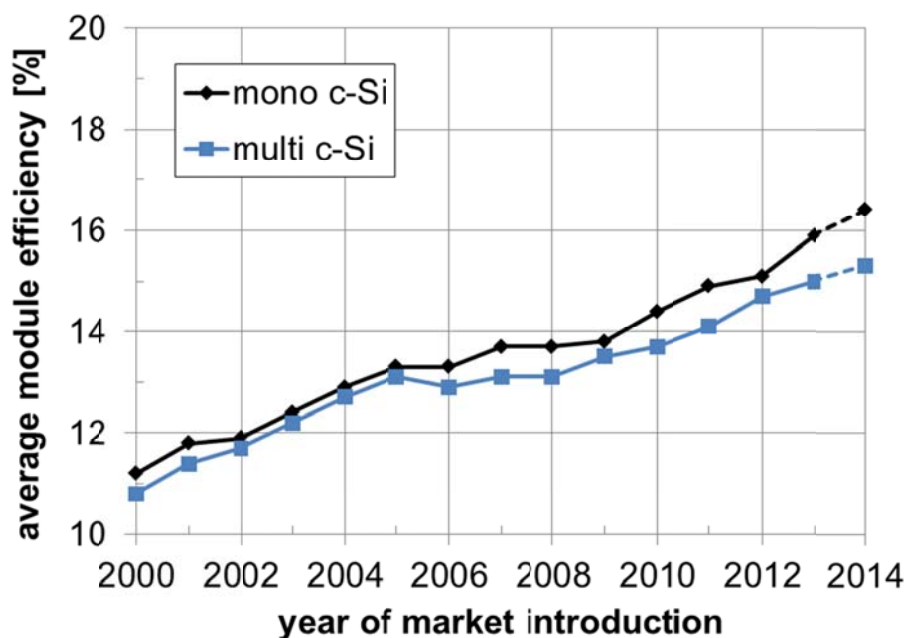
Abbildung 36: Entwicklung der mittleren Wirkungsgrade von PV-Module auf Basis von mono- und multikristallinen Zellen nach dem Jahr der Markteinführung, Daten aus Photon International 2014-02
