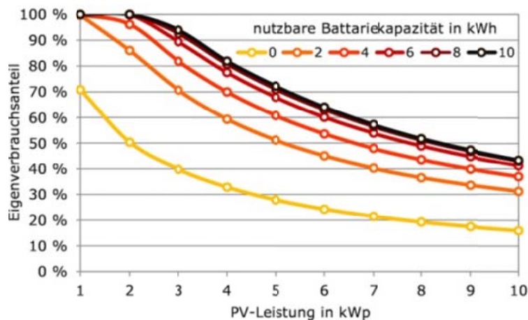
Abbildung 62: Eigenverbrauchsanteil in Abhängigkeit von Batteriekapazität und Leistung des Solargenerators für einen Einfamilienhaushalt mit einem Jahresstromverbrauch von 4.700 kWh. [Quasch]
