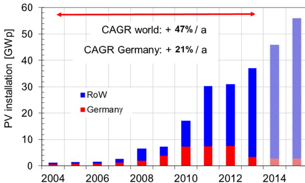
Abbildung 43: Entwicklung des jährlichen PV-Zubaus für Deutschland und die restliche Welt („RoW“) mit Prognosen ab 2014; „CAGR“ steht für die mittlere jährliche Wachstumsrate
