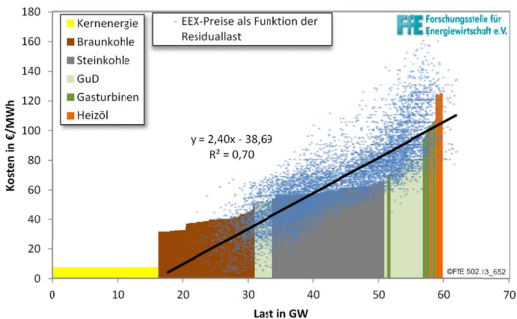
Abbildung 9: Merit Order für das Jahr 2008 und EEX-Preise [Roon]
