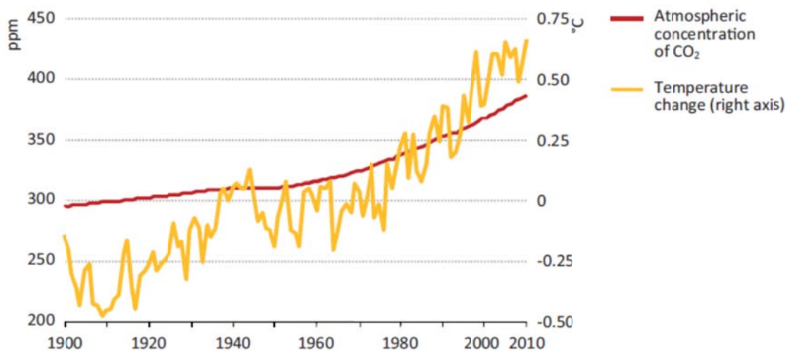
Abbildung 40: Entwicklung der atmosphärischen CO 2 -Konzentration und der mittleren globalen Temperaturveränderung nach dem NASA Global Land-Ocean Temperature Index [IEA2].
