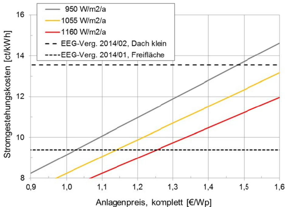
Abbildung 26: Grobe Abschätzung der Stromgestehungskosten für PV-Anlagen unter verschiedenen Einstrahlungsbedingungen
