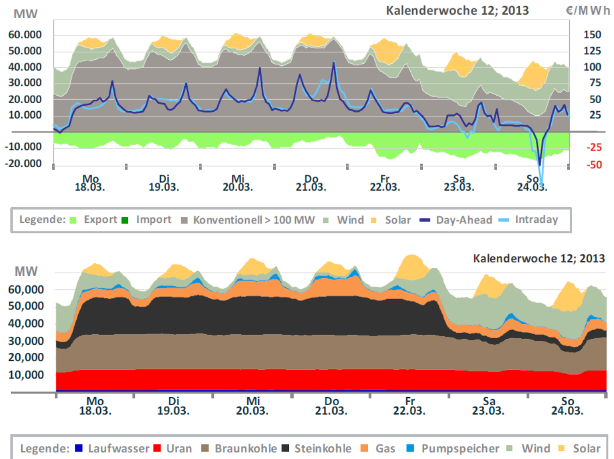
Abbildung 35: Beispiel für den Verlauf von Börsenstrompreisen, konventioneller und regenerativer Stromerzeugung der 12. Kalenderwoche im März 2013 [ISE8]
