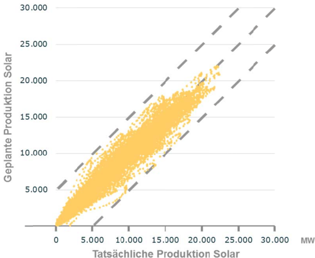
Abbildung 32: Stündliche tatsächliche und geplante Stromproduktion im Jahr 2012 [ISE4]
