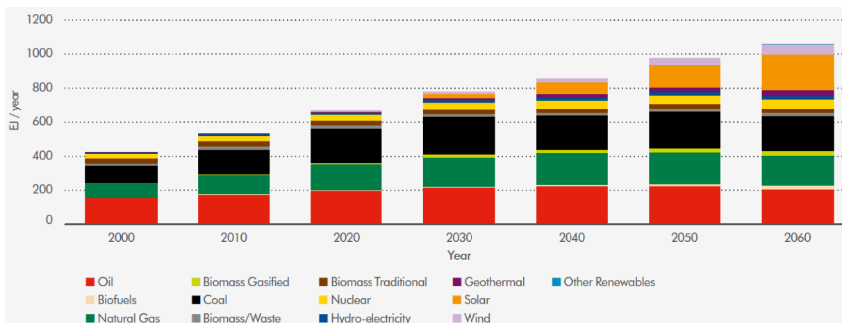
Abbildung 48: Primärenergieverbrauch nach Quellen [Shell]
