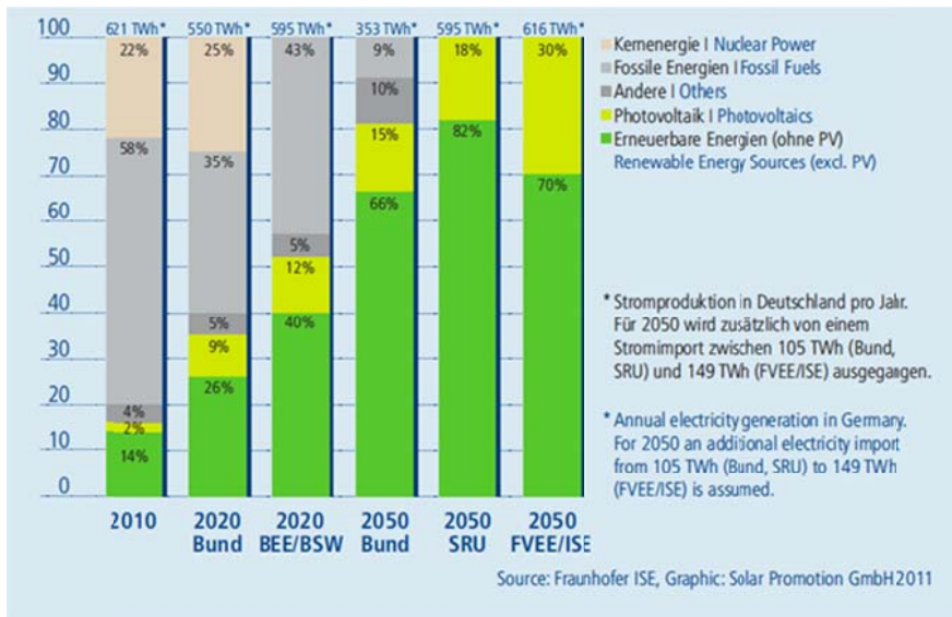
Abbildung 47: Szenarien für die Anteile der Energiequellen an der deutschen Stromproduktion [ISE3]
