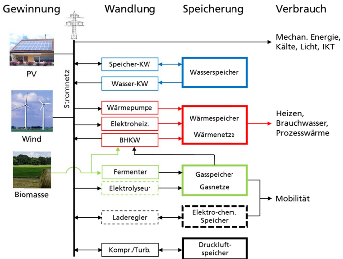
Abbildung 44: Vereinfachte schematische Darstellung eines Erneuerbaren Energiesystems mit den wichtigsten stromnetzgebundenen Bausteinen der Kategorien Gewinnung, Wandlung, Speicherung und Verbrauch; IKT: Informations- und Kommunikationstechnik; gestrichelte Kästen: zur Zeit noch sehr geringe Leistungen/Kapazitäten verfügbar
