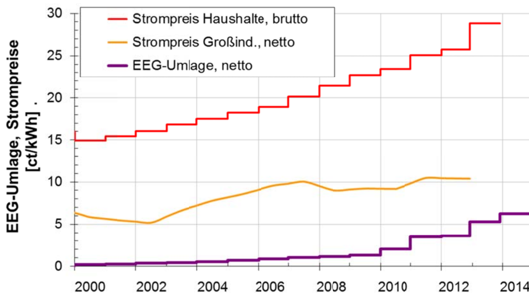
Abbildung 21: Entwicklung von Brutto-Strompreisen für Haushalte, von Netto-Strompreisen für industrielle Großabnehmer [BMWi1] und Entwicklung der EEG-Umlage; die Brutto-Strompreise der Haushalte bestehen heute zur Hälfte aus Steuern und Abgaben
