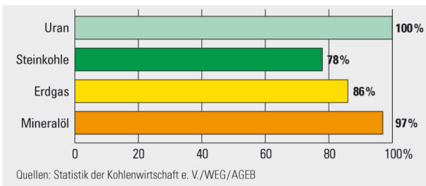
Abbildung 50: Abhängigkeit Deutschlands von Energierohstoffimporten 2011
