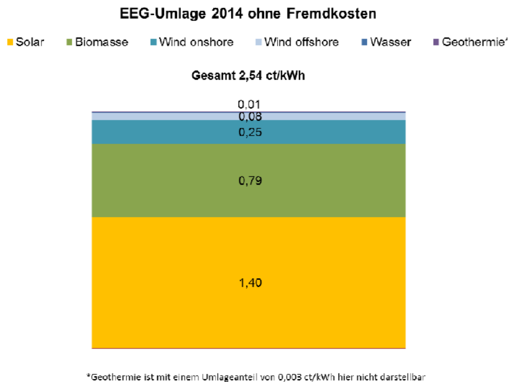
Abbildung 16: Bestandteile der EEG-Umlage 2014 ohne Fremdkosten [BEE1]
