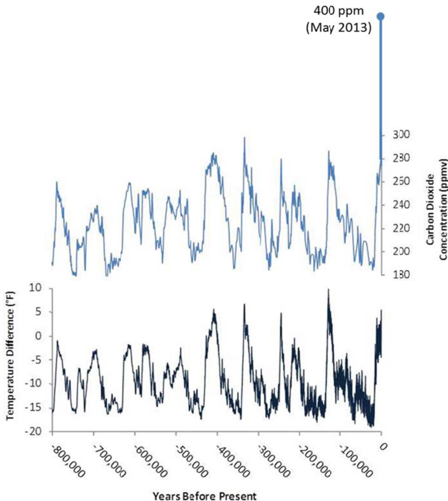
Abbildung 41: Schätzungen der atmosphärischen CO 2 -Konzentration und der Temperatur in der Antarktis auf Basis von Eisbohrkernen [EPA], CO 2 -Konzentration für 2013 wurde hinzugefügt
