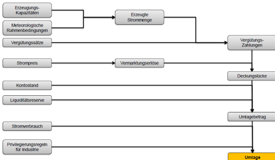
Abbildung 14: Übersicht zu Einflussfaktoren und Berechnung der EEG-Umlage [ÖKO]
